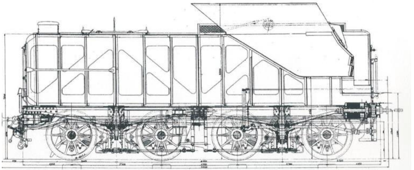
Zeichnung Aussenansicht des Tenders 37 m/cub
