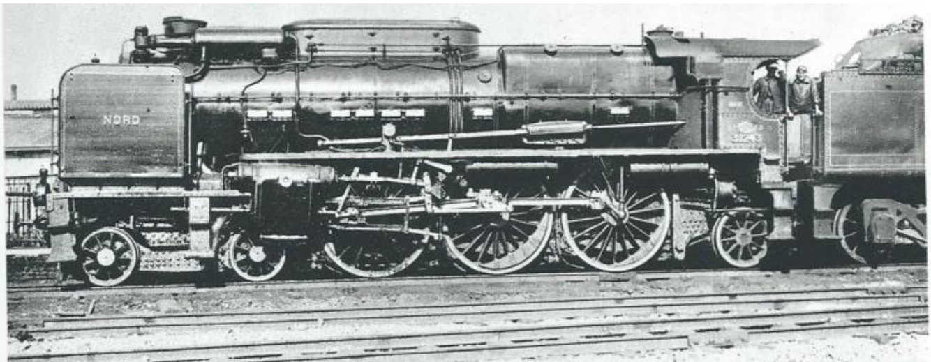
sehr seltene Aufnahme der NORD no 3.1243 typ "CERCEUIL" mit Windleitblechen und Réchauffeur (wie Art.no. 2269/3)
