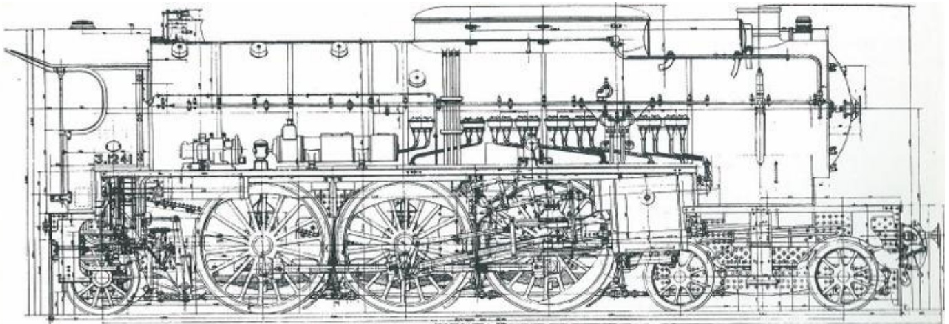
Zeichnung Aussenseite der Pacific NORD no 3.1241 mit verkleideten Domen "CERCEUIL" ohne Windleitbleche (wie Art.no. 2269/2)
