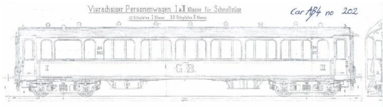
GB (Gotthardbahn) AB4 no 202, der frühen, blauen Ausführung (Abteilseite)
